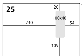
C4 pose (229x324 mm) tværstillet rude
