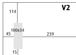
C4M (229x318 mm) tværstillet rude
