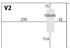
EC4 pose (229x312 mm) tværstillet rude
